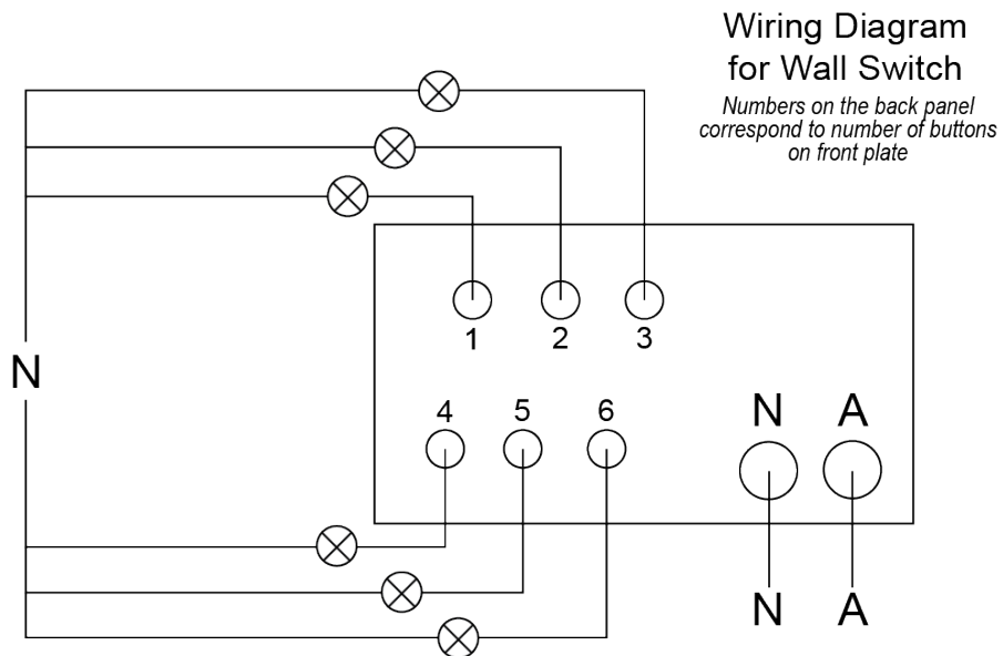
T-R30 Wiring Diagram
