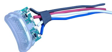
PCBKIT-S
